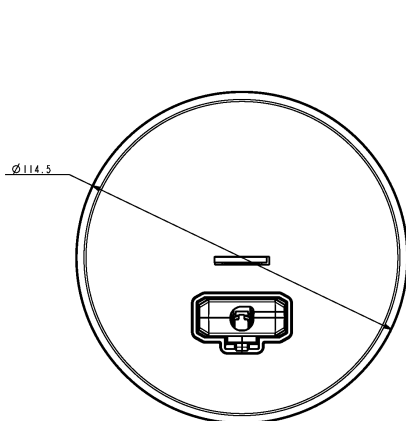
Måttritning
