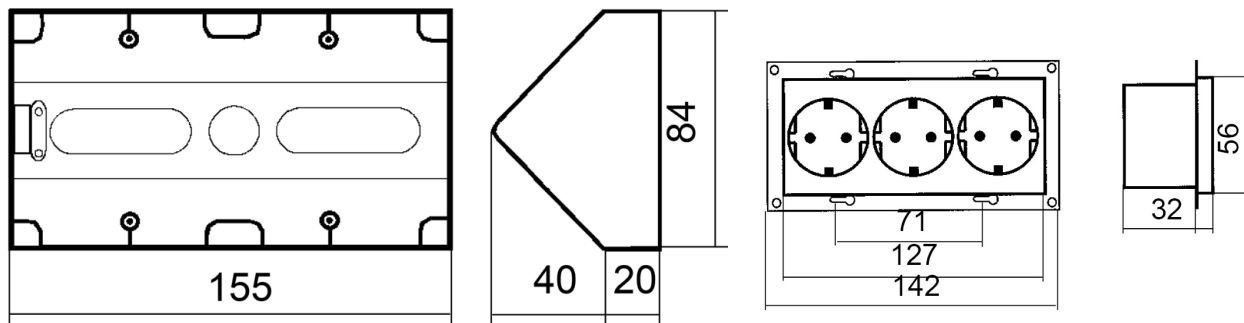
Måttritning
