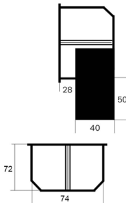
Måttritning
