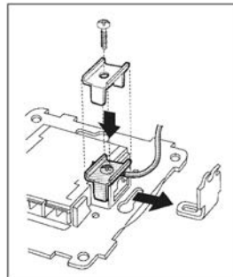
Montering av jordbleck.
