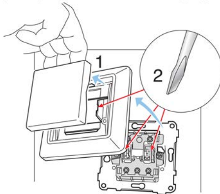
Montering av impulsfjäder.
